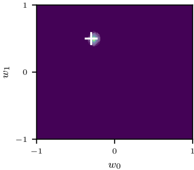
prior/posterior
